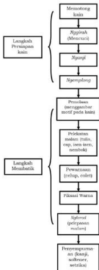
Gambar 2 – Bagan Alir Proses Produksi Industri Batik
