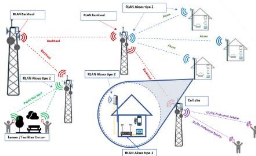
Gambar 2. Ilustrasi topologi RLAN untuk Akses dan Backhaul
