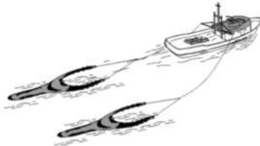
Gambar pukat hela dasar udang
