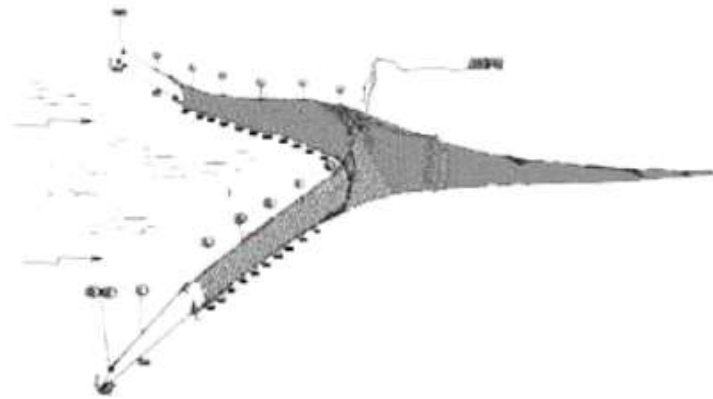
Gambar pukat labuh
