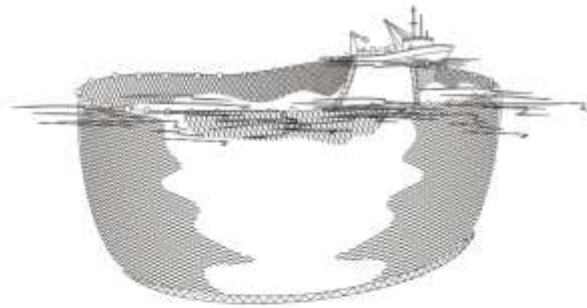
Gambar pukat cincin dengan satu kapal
