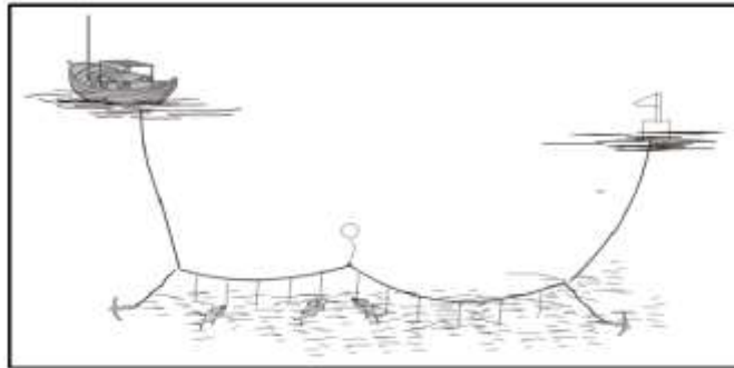
Gambar rawai dasar
