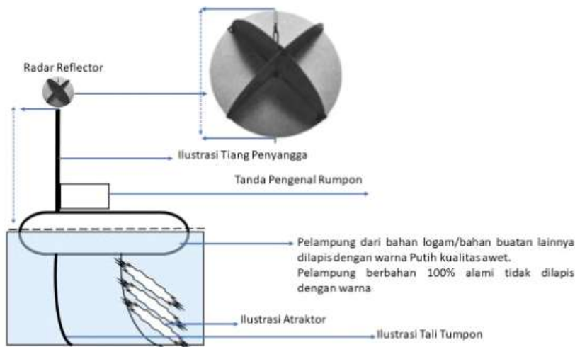
TANDA PENGENAL RUMPON DAN RADAR REFLEKTOR
