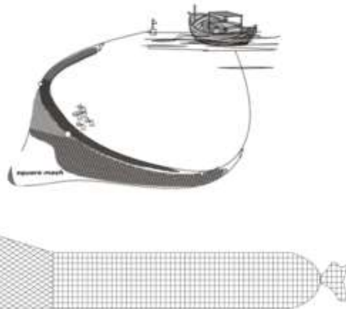
Gambar jaring tarik berkantong dan sketsa mata jaring kantong berbentuk persegi
