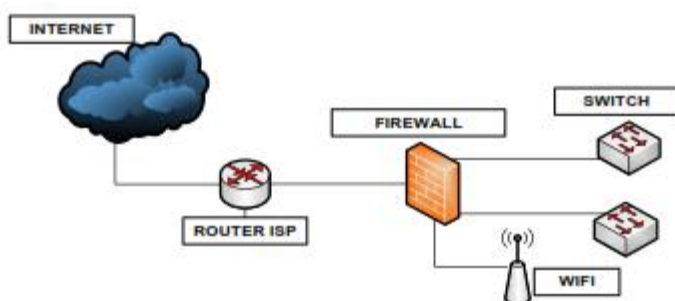
Penempatan firewall
