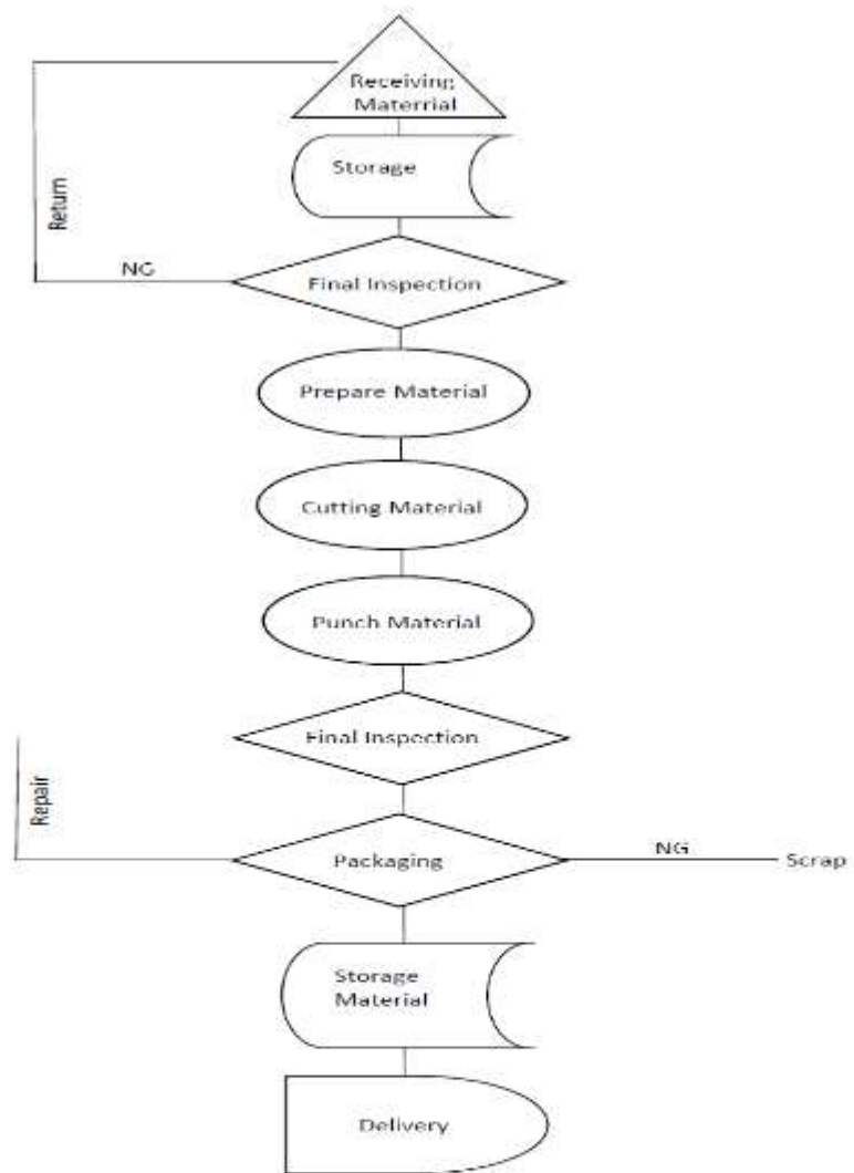
Gambar 3 – Bagan Alir Produksi Silencer
