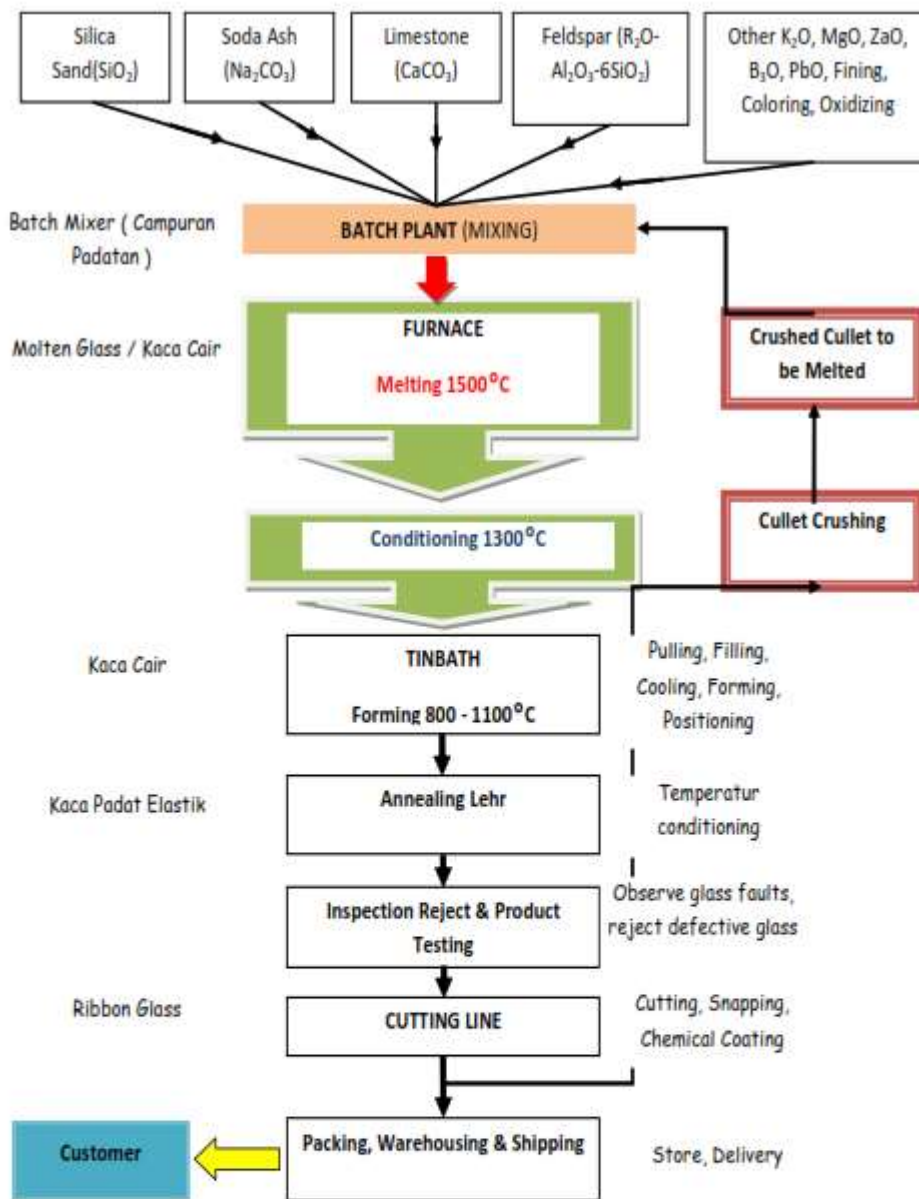
Gambar 4 – Diagram Alir Proses Produksi Kaca Lembaran.
