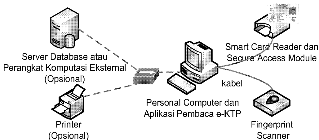
Gambar 1. Perangkat Pembaca dan/atau Penulis KTP Elektronik (Terpisah)
