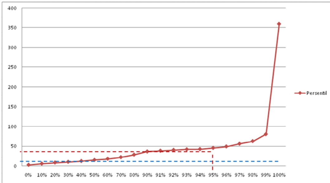
Gambar IV.20 Grafik Curah Hujan Persenti 0% - 100%
