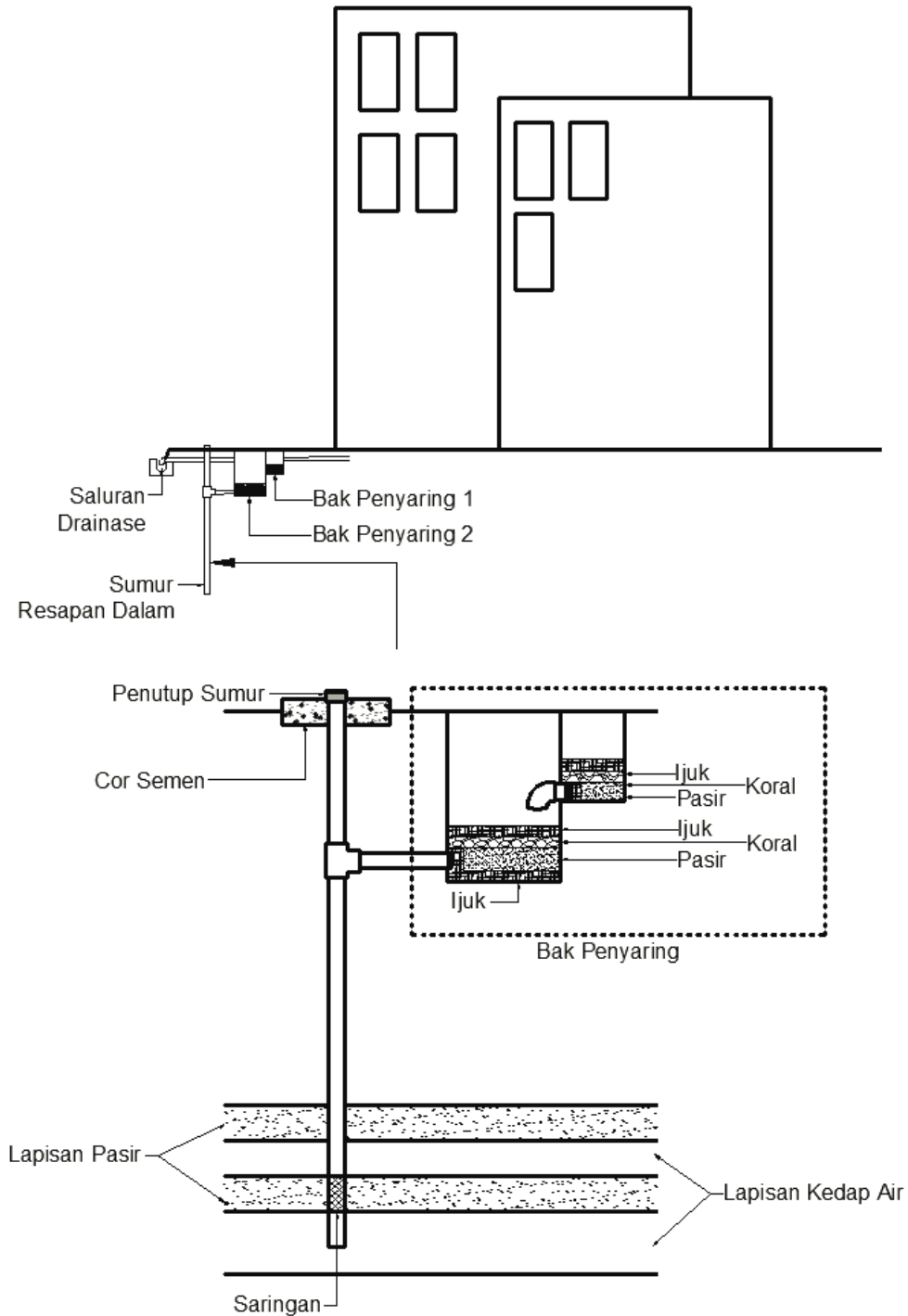
Gambar IV.10 Ilustrasi Sistem Sumur Resapan Dalam
