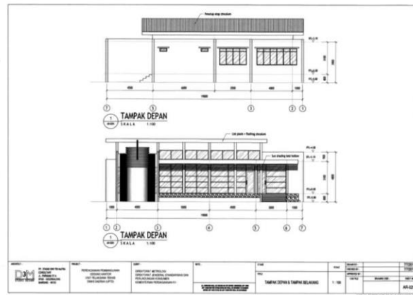
Gambar 7 Tampak Depan Gedung Kantor dan Laboratorium Unit Metrologi Legal Kabupaten/Kota
