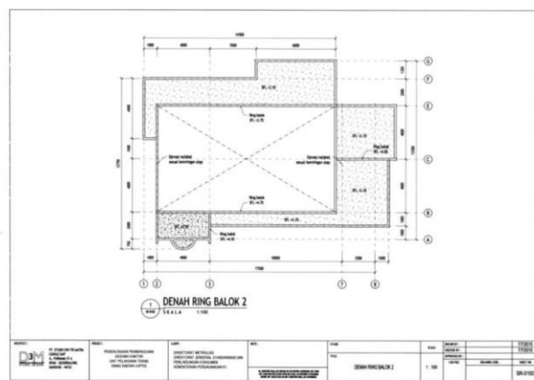
Gambar 24 Denah Ring Balok 2 Gedung Kantor dan Laboratorium Unit Metrologi Legal Kabupaten/Kota
