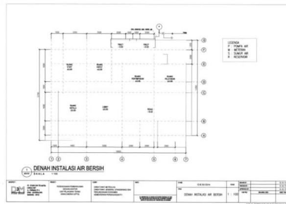
Gambar 19 Denah Instalasi Air Bersih Gedung Kantor dan Laboratorium Unit Metrologi Legal Kabupaten/Kota
