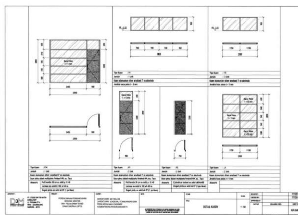
Gambar 15 Lanjutan Detail Kusen Gedung Kantor dan Laboratorium Unit Metrologi Legal Kabupaten/Kota
