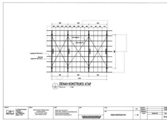
Gambar 26 Denah Konstruksi Atap Gedung Kantor dan laboratorium Unit Metrologi Legal Kabupaten/Kota
