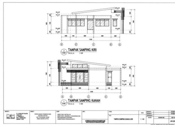
Gambar 8 Tampak Samping Kiri dan Kanan Gedung Kantor dan Laboratorium Unit Metrologi Legal Kabupaten/Kota
