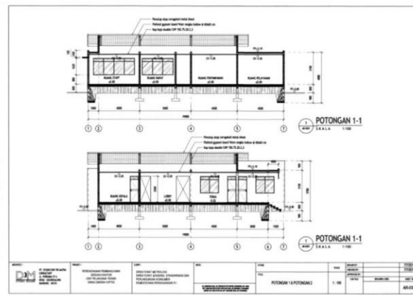
Gambar 9 Potongan 1-1 Gedung Kantor dan Laboratorium Unit Metrologi Legal Kabupaten/Kota
