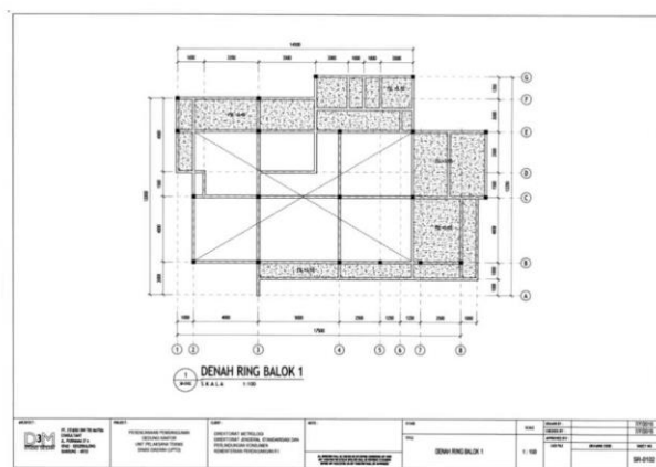
Gambar 23 Denah Ring Balok 1 Gedung Kantor dan Laboratorium Unit Metrologi Legal Kabupaten/Kota
