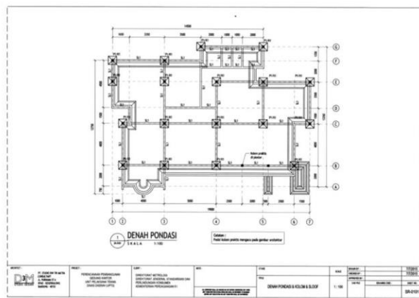
Gambar 22 Denah Pondasi Gedung Kantor dan Laboratorium Unit Metrologi Legal Kabupaten/Kota
