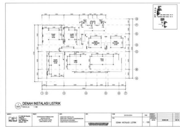
Gambar 21 Denah Instalasi Listrik Gedung Kantor dan Laboratorium Unit Metrologi Legal Kabupaten/Kota
