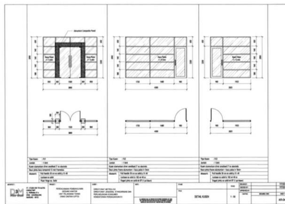
Gambar 14 Detail Kusen Gedung Kantor dan Laboratorium Unit Metrologi Legal Kabupaten/Kota
