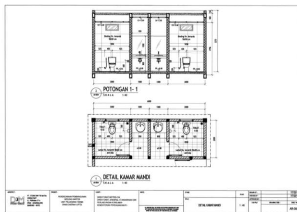
Gambar 18 Detail Kamar Mandi Gedung Kantor dan Laboratorium Unit Metrologi Legal Kabupaten/Kota
