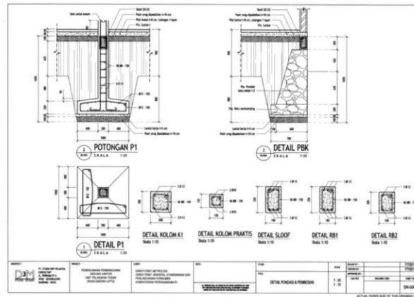
Gambar 25 Detail Pondasi & Pembesian Gedung Kantor dan Laboratorium Unit Metrologi Legal Kabupaten/Kota
