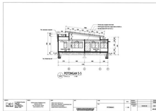
Gambar 11 Potongan 5-5 Gedung Kantor dan Laboratorium Unit Metrologi Legal Kabupaten/Kota
