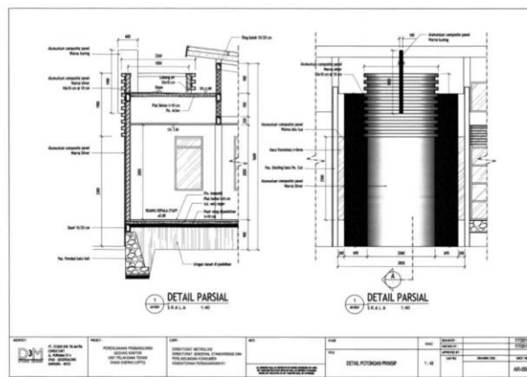
Gambar 17 Detail Potongan Prinsip Gedung Kantor dan Laboratorium Unit Metrologi Legal Kabupaten/Kota
