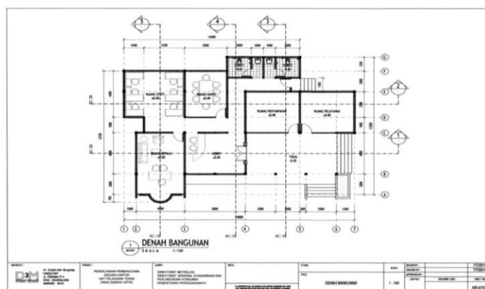
Gambar 5 Denah Bangunan Gedung Kantor dan Laboratorium Unit Metrologi Legal Kabupaten/Kota
