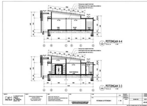
Gambar 10 Potongan 3-3 Gedung Kantor dan Laboratorium Unit Metrologi Legal Kabupaten/Kota
