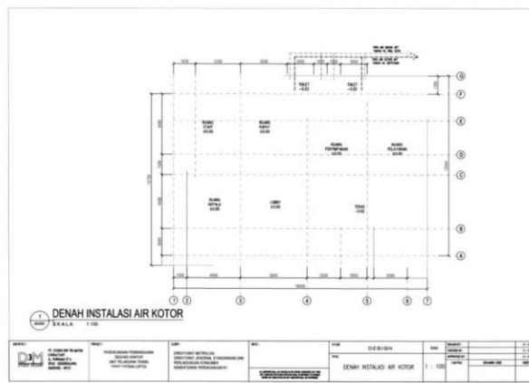
Gambar 20 Denah Instalasi Air Kotor Gedung Kantor dan Laboratorium Unit Metrologi Legal Kabupaten/Kota
