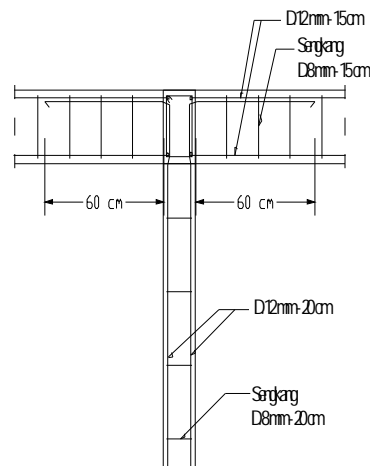
DETAIL L.B. KOLOM BERTENGAH DENGAN RING BALOK
