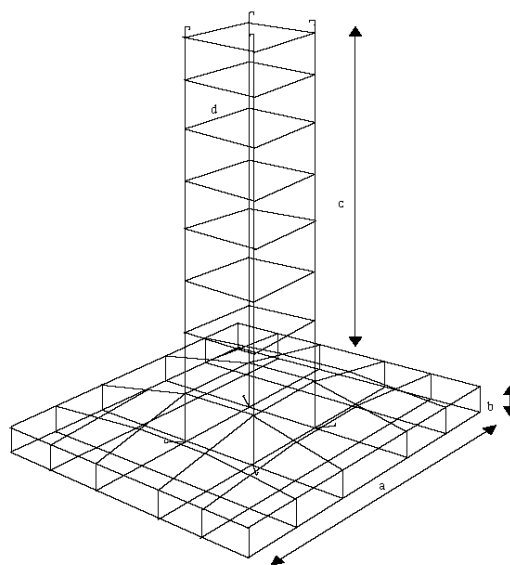
(b) Rangkaian besi
