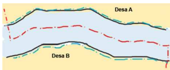
Gambar 1. Garis putus-putus berwarna merah menunjukkan garis batas pada as sungai dan warna biru menunjukkan garis batas pada tepi sunaai.
