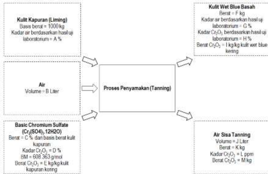
Gambar 2 – Diagram Input dan Output Proses Penyamakan
