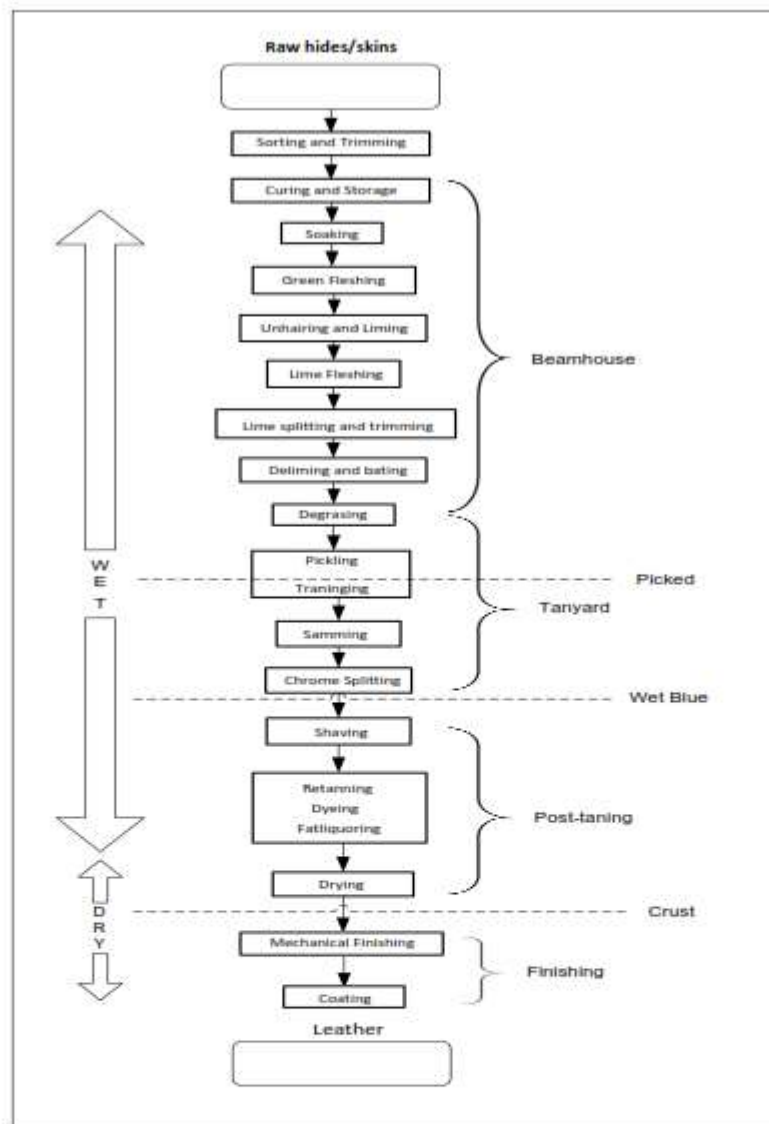
Gambar 6 - Diagram Alir Proses Penyamakan Kulit
